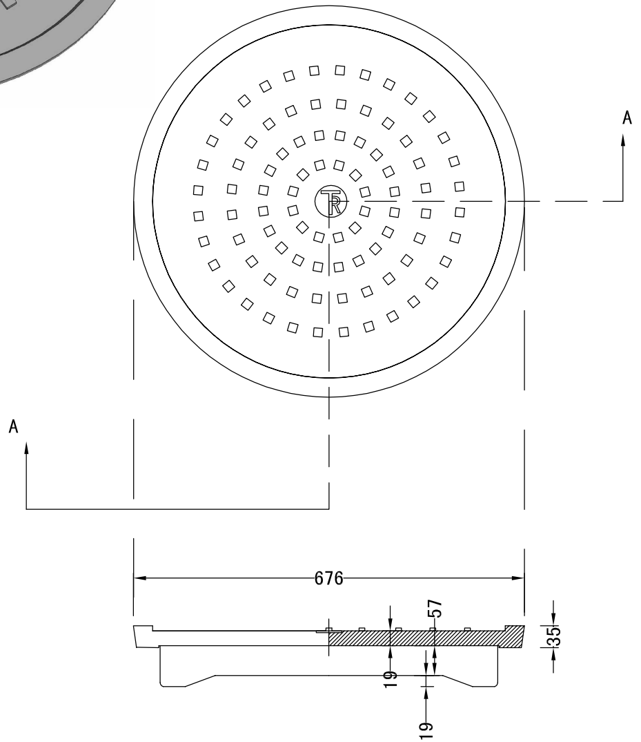
SECTION A-A
