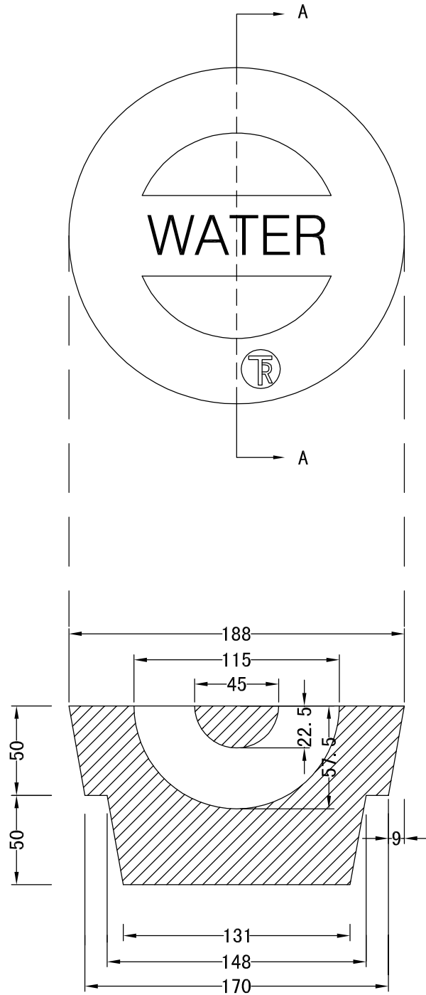
SECTION A-A
